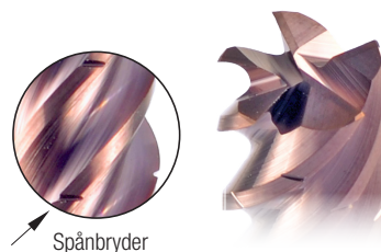
Spånbryder
